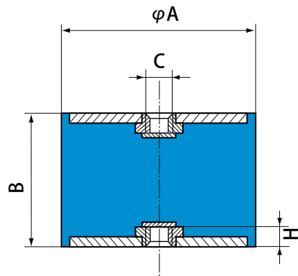
双螺孔
