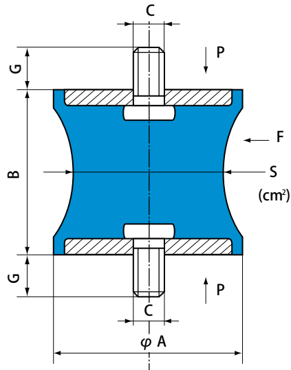
空头螺柱型
