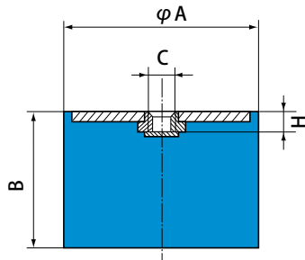
一端螺纹孔
