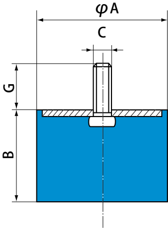
单边螺柱
